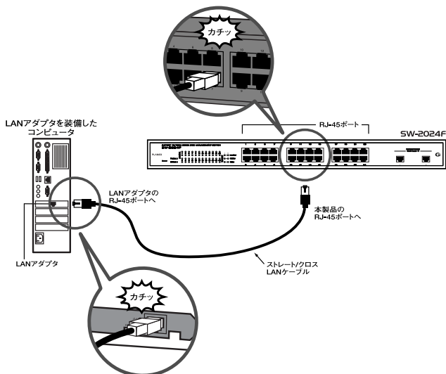
図2-5 RJ-45ポートを使用した接続
