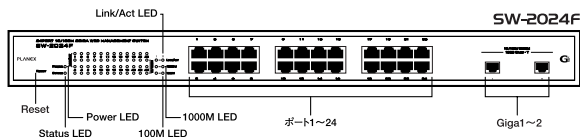
図1-1 前面パネル
