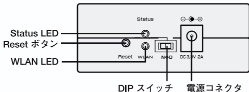
図1-2 Mini-UWFの背面図
