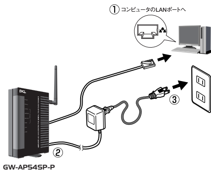
図3-1 GW-AP54SP-P 機器の接続
