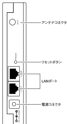
図1-3 GW-AP54SP-P背面図
