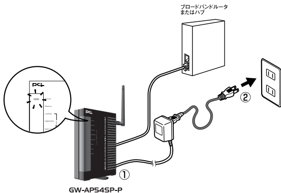
図2-2 GW-AP54SP-P 電源の接続
