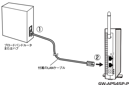
図2-1 GW-AP54SP-P ネットワーク機器との接続
