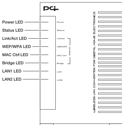
図1-2 GW-AP54SP-P前面図
