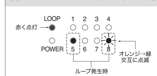
(例) LANポート5と8でループが発生した時のLED状態
