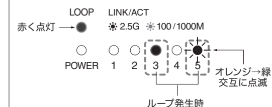
(例) LANポート3と5でループが発生した時のLED状態
