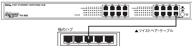
図2-2 他のハブとのカスケード接続
