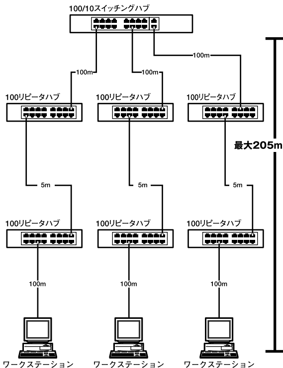
図C-3 スイッチングハブを併用したカスケード接続の制限
