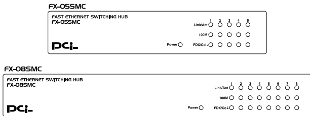
図1-1 前面パネル
