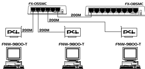
図1-5 フローコントロール対応 100Base-TX ネットワーク構築例
