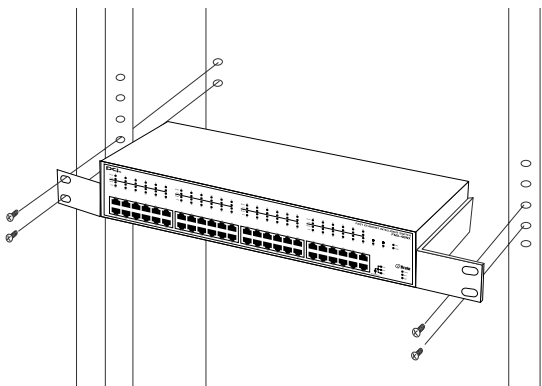
図2-3 ラックへの取り付け
