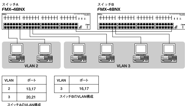
図1-8 「IEEE802.1Qベース」VLAN構成例
