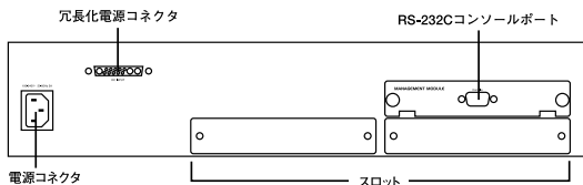
図1-2 FMX-48NX 背面図
