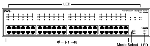
図1-1 FMX-48NX 前面図
