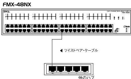
図2-6 他のハブとのカスケード接続
