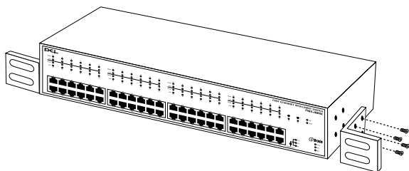
図2-2 ラックマウント用金具の取り付け
