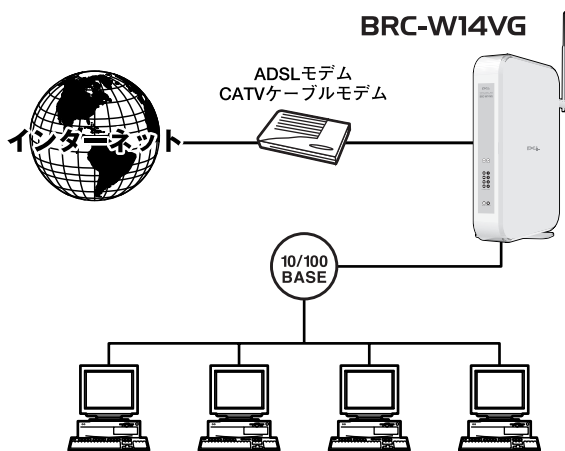
図1-1 接続図
